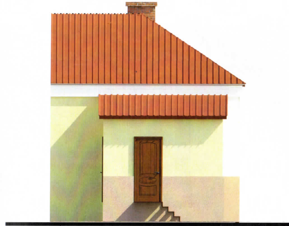
Фасад в осях В-А
